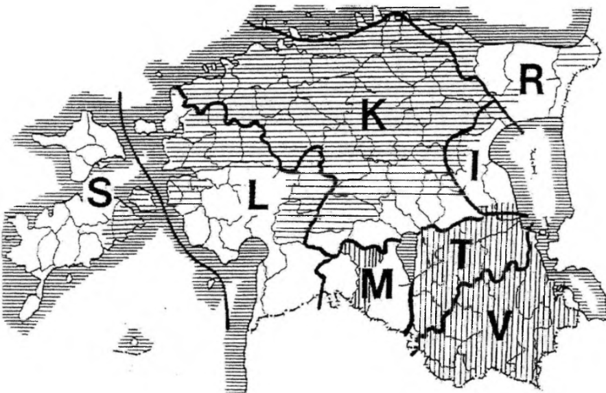
Pika \delta diftongistumine (—) ja kõrgenemine (|) kolmandavärtelistes sõnades eesti murretes (Teras 2003).
