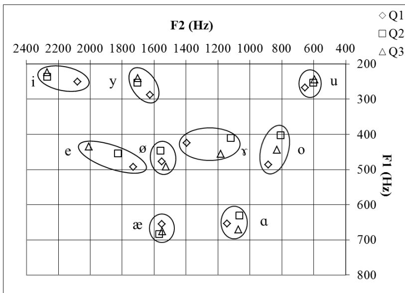
Loetud kõne esma-, teise- ja kolmanda-väeteliste sõnade täishäälikud formantruumis (Eek, Meister 1998)
