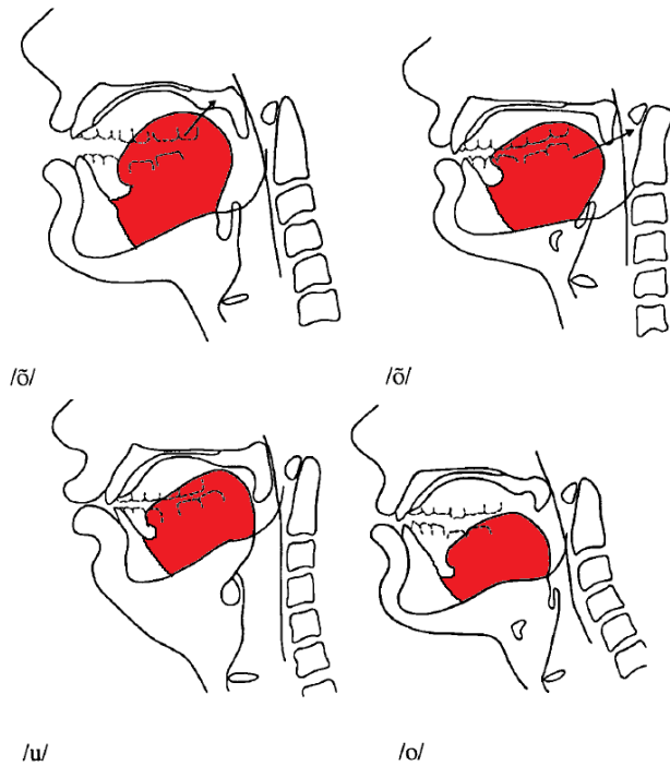
Keele asendid täishäälikute /õ/, /u/ ja /o/ hääldamisel (Eek 2008: joonis 2.8; Liiv 1961)
