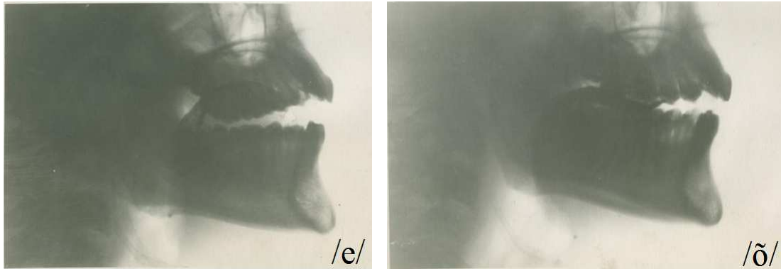
Röntgenogrammid täishäälikutest /e/ ja /õ/ (keelejuht J. Paalma) (TÜ eesti murrete ja sugulaskeelte arhiiv, fotod PF0004-038, PF0004-006).
