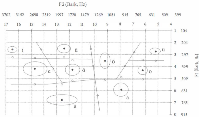
Täishäälikute sihtväärtused standardhälvetega ja täishäälikukategooriate vahelised piirid tajuruumis (Eek, Meister 1994).
