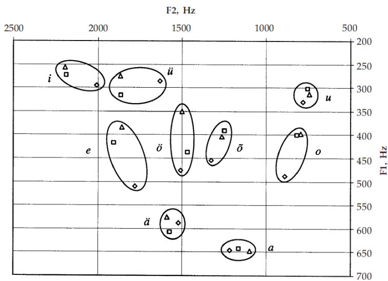
Muhu vanemate keelejuhtide esmävälteliste (□), teisevälteliste (◇) ja kolmandavälteliste (△) sõnade täishäälikud formantruumis (Niit 2007).
