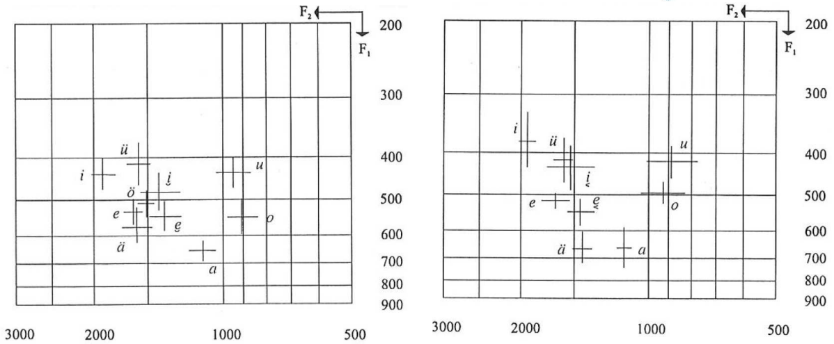
Võru murde lühikesed täishäälikud 1. silbis (vasakul) ja 2. silbis (paremal) (Parve 2000).
