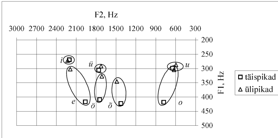
Võru kolme meeskeelejuhi keskkõrged ja kõrged vokaalid teisevältelistes (täispikad) ja kolmandavältelistes (ülipikad) sõnades loetud kõnes (Teras 2003).
